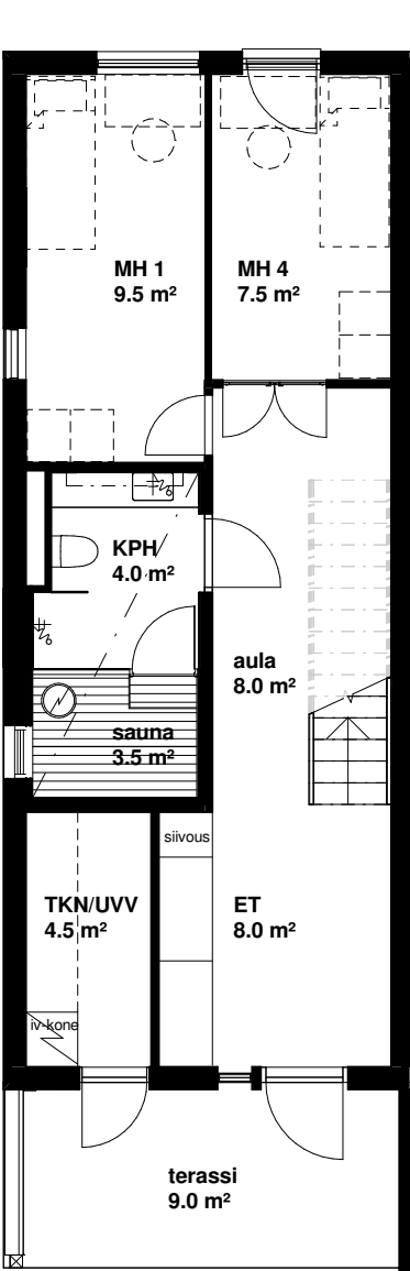
▲ Pohjakuva 1 krs lisämakuuhuoneilla
